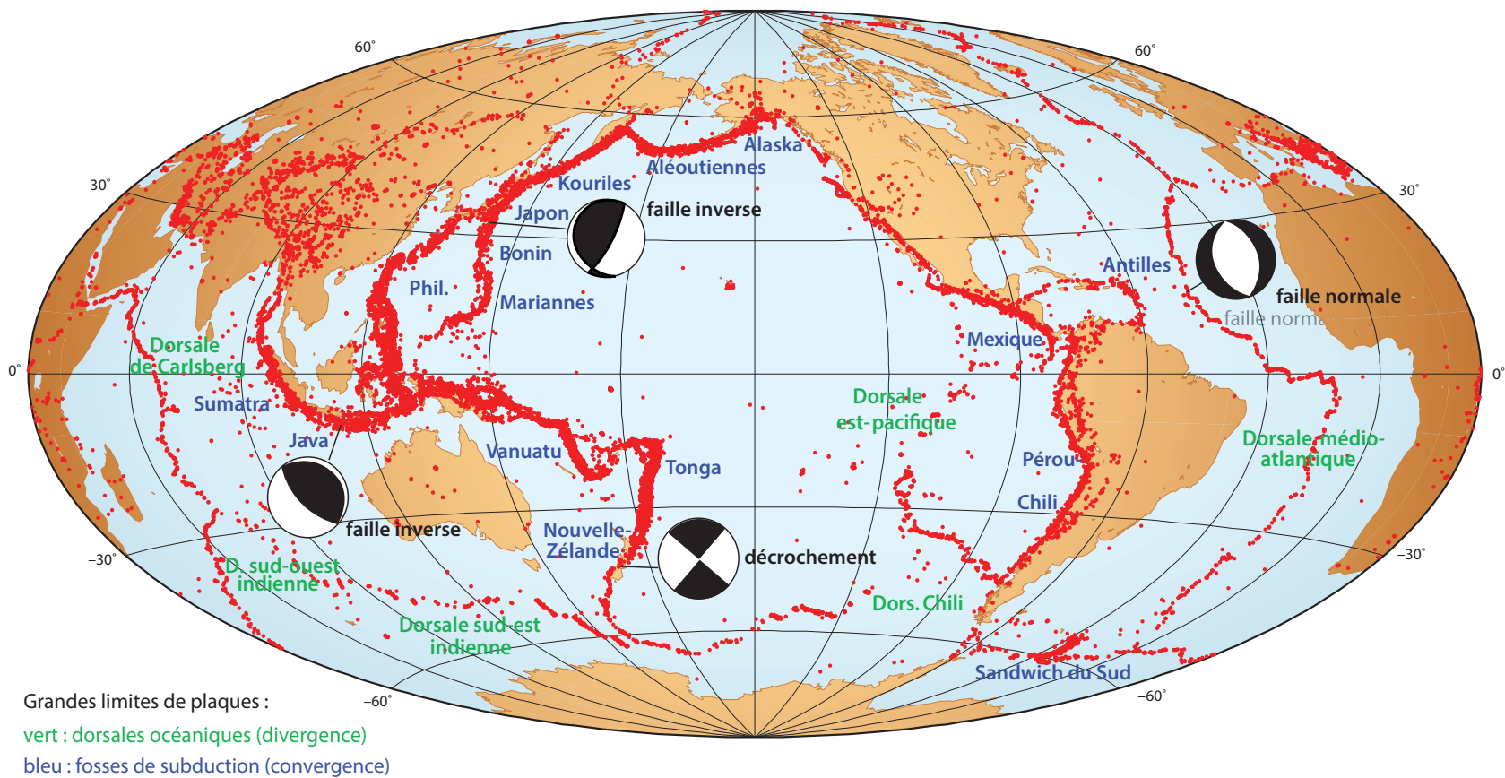
Figure 1 : carte de la sismicité mondiale (in Renart et al., 2016)
