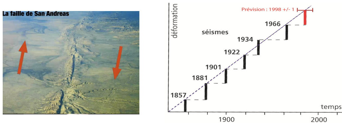
Figure 13 : récurrence et prévision d'un séisme sur la faille de San Andreas (Californie)
