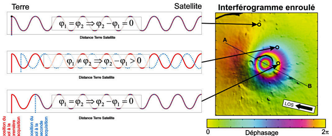
Figure 10.c : conséquences de la longueur d'onde utilisée par le satellite
