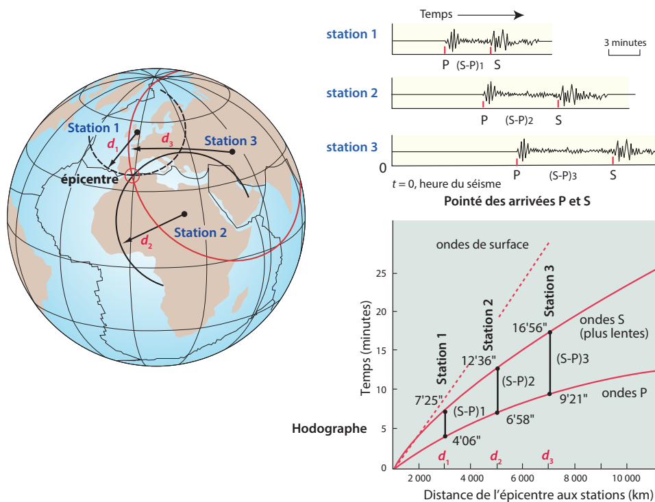
Figure 6.17 Principe de la détermination des épicentres (et hypocentres) par la méthode S-P.
